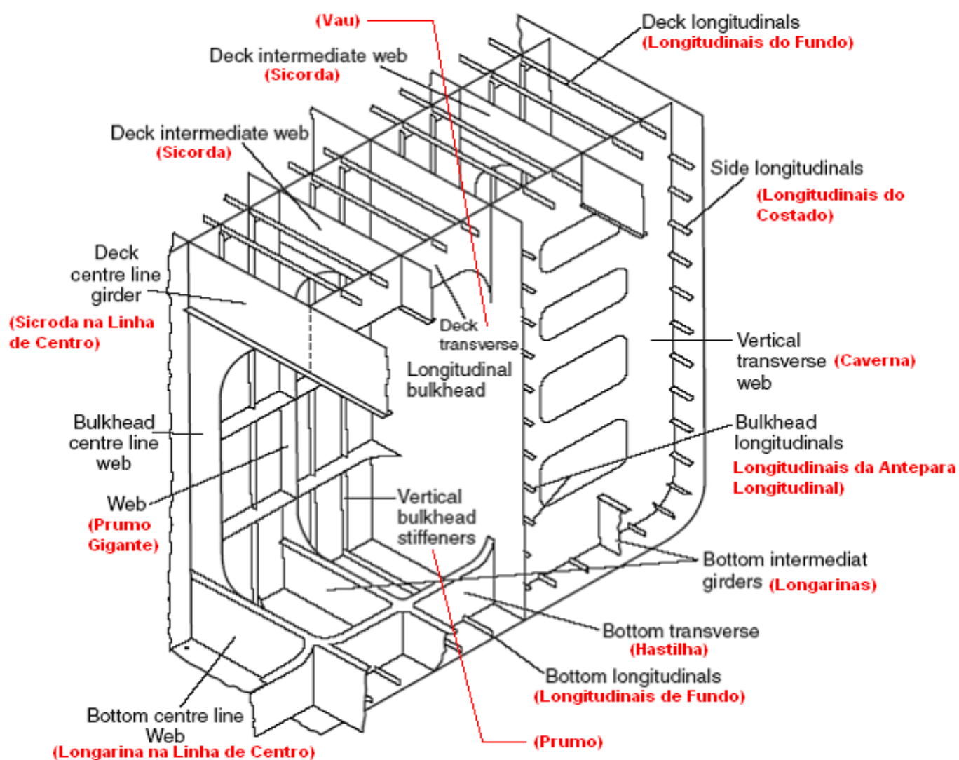
Figura 2 – Compartimento interno de um tanque
