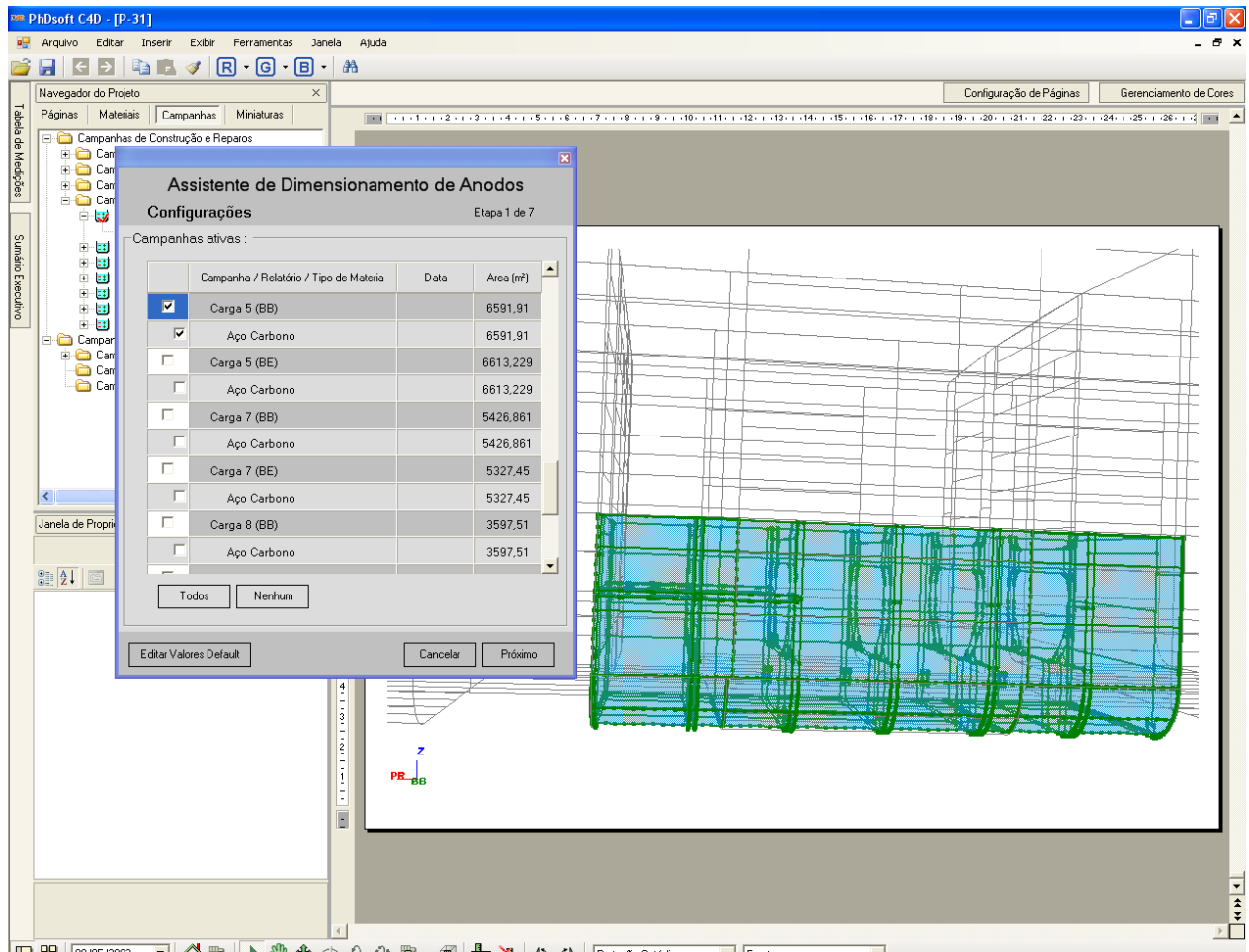
Figura 6 – Área de proteção catódica em destaque e janela do assistente de dimensionamento de anodos aberta
