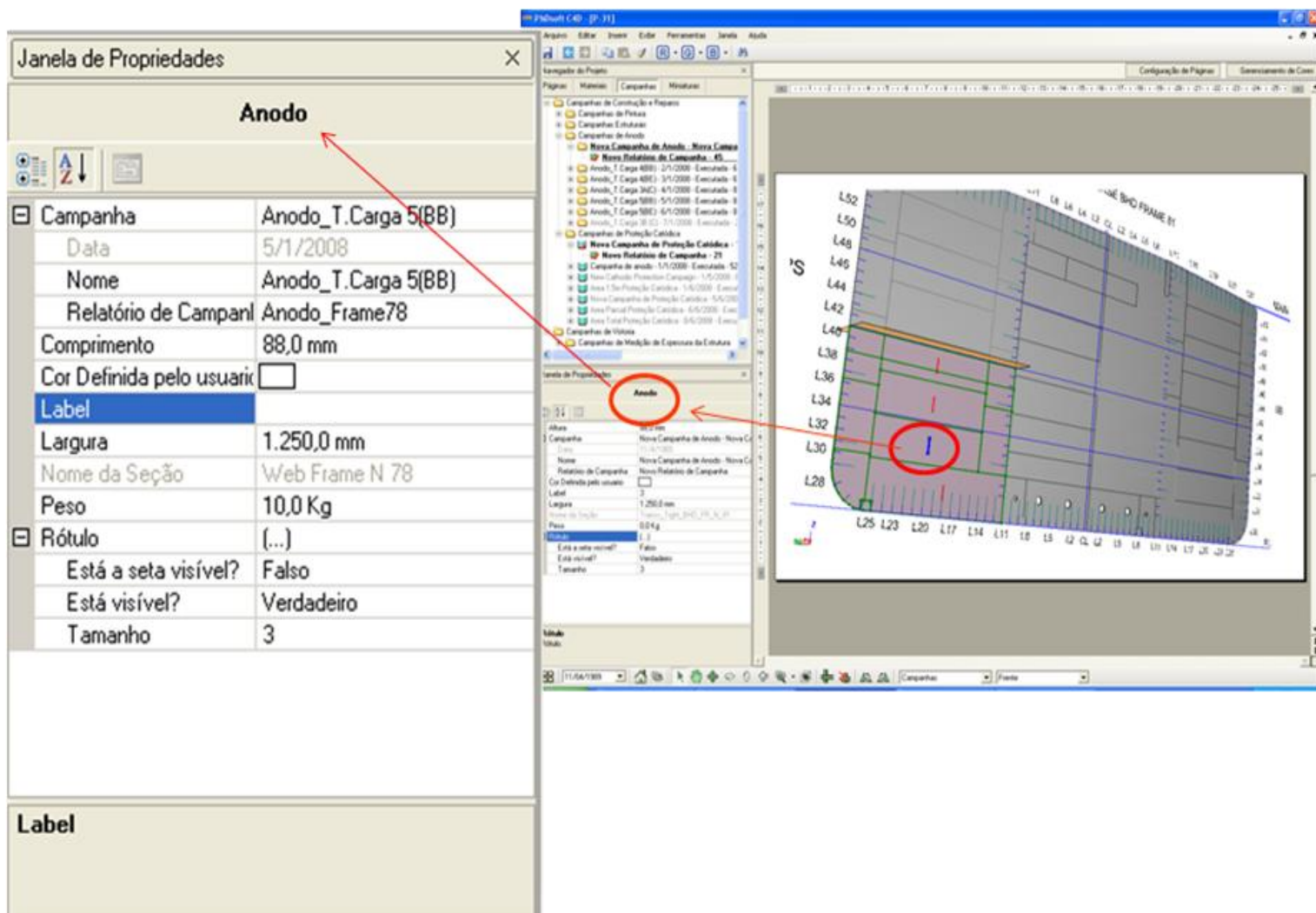
Figura 20 – Visualização de informações sobre o anodo na “Janela de Propriedades” além das informações sobre o tanque que está sendo protegido catodicamente
