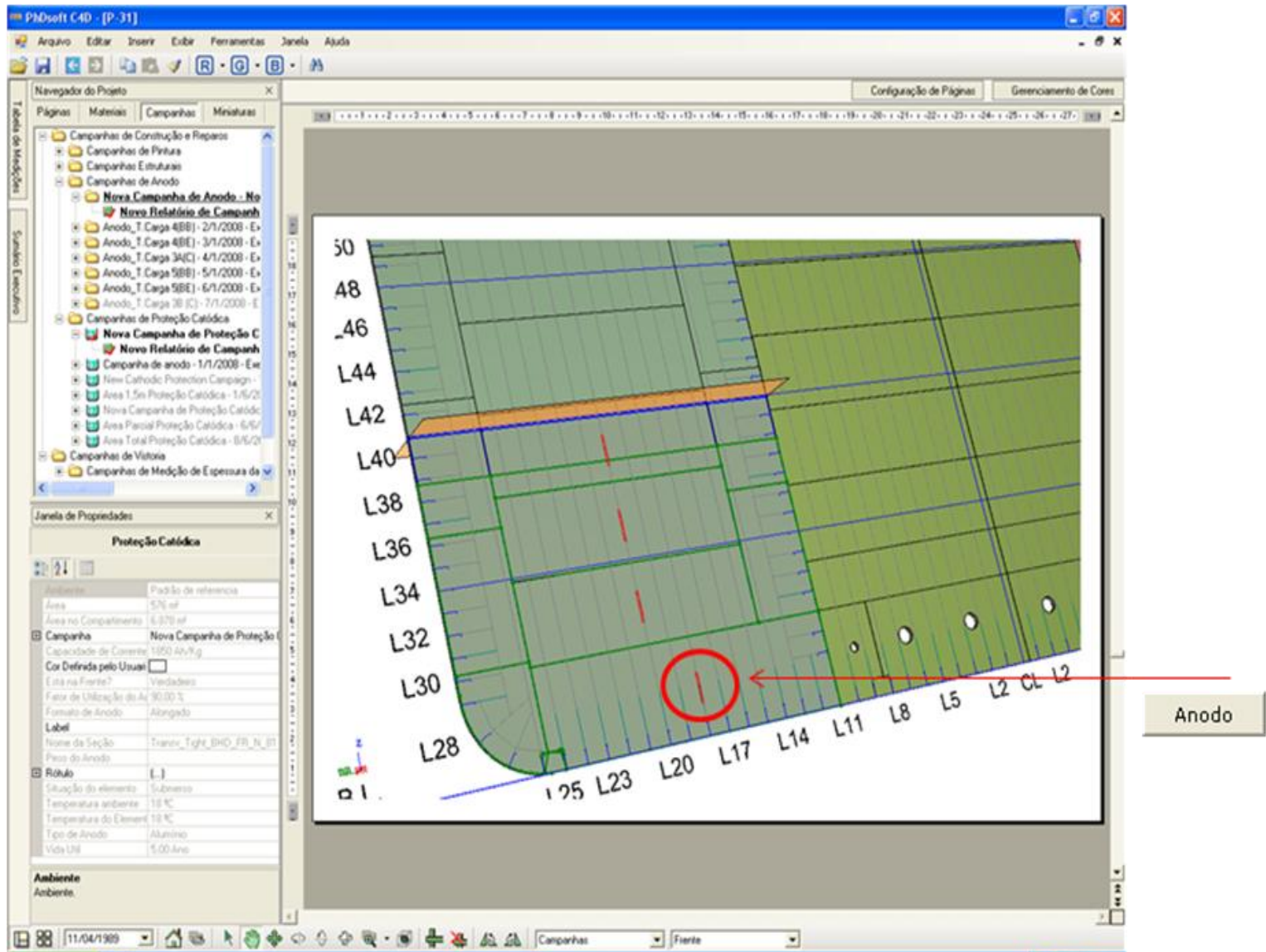
Figura 19 – Visualização dos anodos distribuídos em uma das cavernas do tanque. Logo acima dos anodos pode-se verificar a linha do plano auxiliar (na cor laranja) que indica o limite superior da área a ser protegida catódicamente
