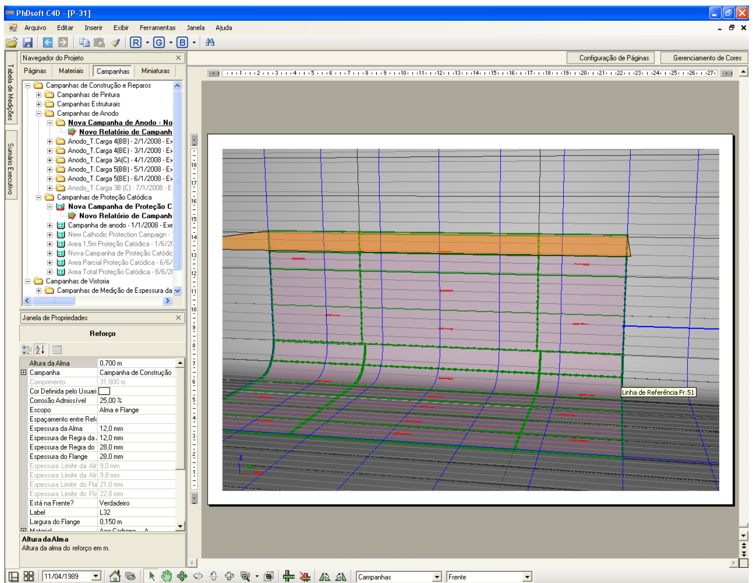
Figura 18 – Visualização dos anodos distribuídos em um dos costados e fundo do tanque. Logo acima dos anodos pode-se verificar a linha do plano auxiliar (na cor laranja) que indica o limite superior da área a ser protegida catodicamente
