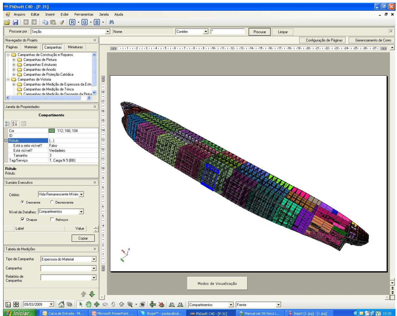
Figura 1 – O modelo da plataforma e seus compartimentos (em diversas cores para distinção das regiões entre tanques)
