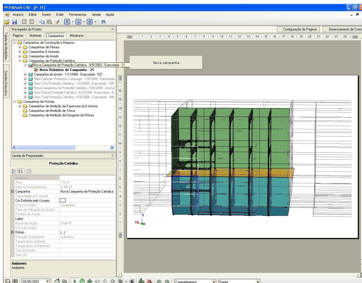
Figura 4 – Delimitação da área a ser protegida (na cor azul abaixo) e criação da nova campanha de proteção catódica para início do dimensionamento dos anodos
